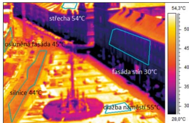
Obr. 7.1.b: Osluněné střechy mají teplotu až 54 °C, dlažba náměstí až 55 °C a fasády domů 45 °C a fasády ve stínu 30 °C
